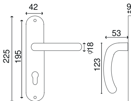
Lacanau 195 Assemblage par vis relieuses
