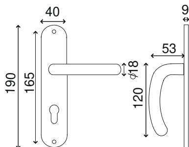
Lacanau 165 Assemblage par vis relieuses
