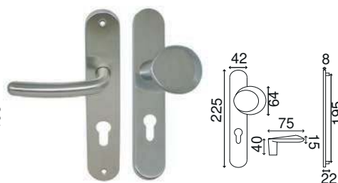
Ensemble palière AMANDE LACANAU
