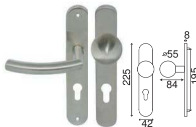
Ensemble palière BOULE LOUPIAC
