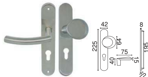
Ensemble palière AMANDE LOUPIAC
